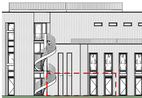
Zuidgevel
