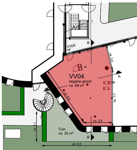
Begane grond
